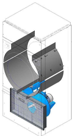
IMPIANTO ASPIRAZIONE SUCTION SYSTEM
