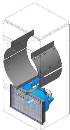
IMPIANTO ASPIRAZIONE SUCTION SYSTEM
